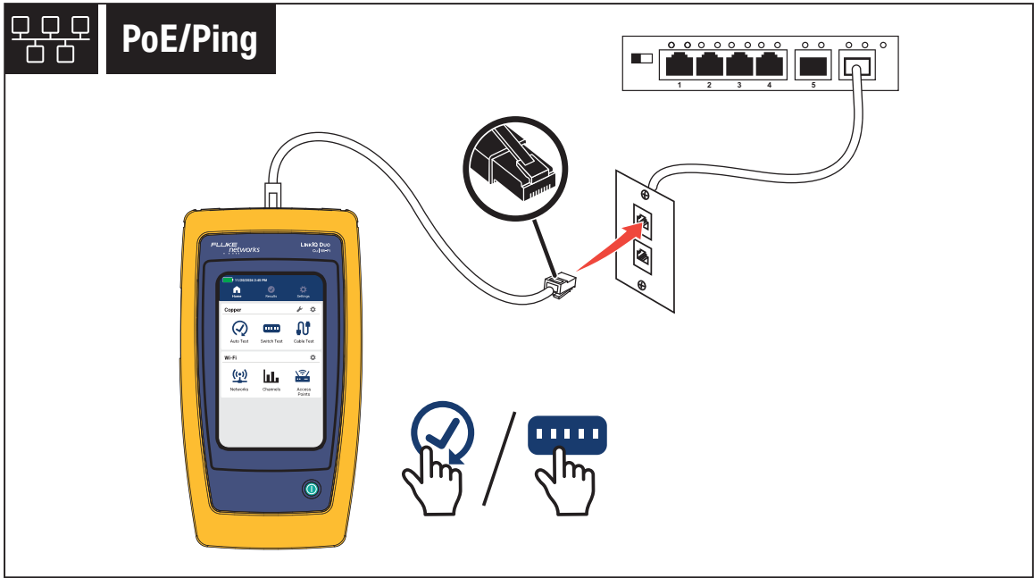
图 2. 交换机测试设置
