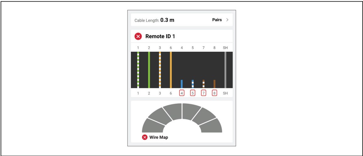
图 5. 开路线对
